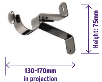
A-Frame Bracket
