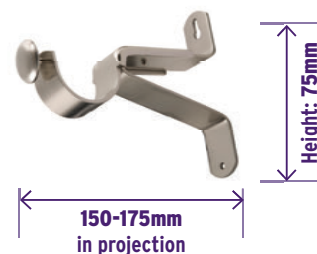
A-Frame Bracket
